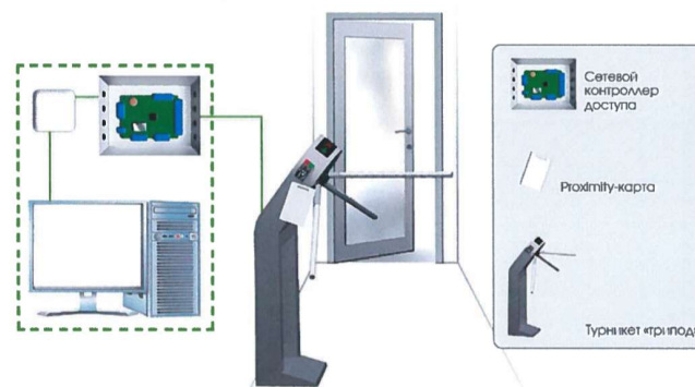
Сетевой контроллер доступа на КПП
